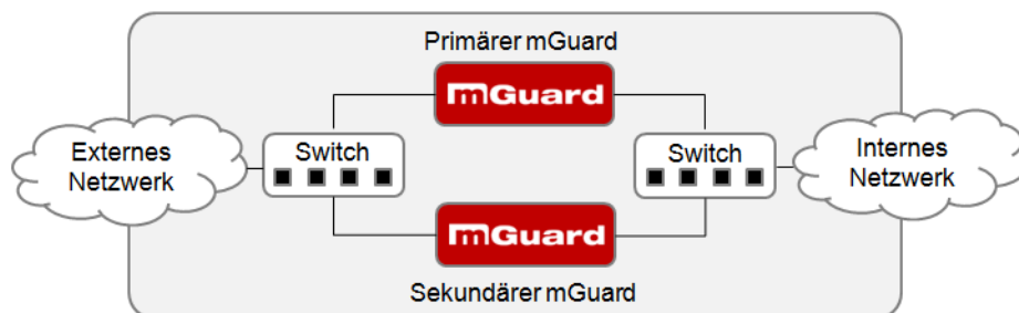
Bild 17-1 Firewall-Redundanz (Beispiel)
