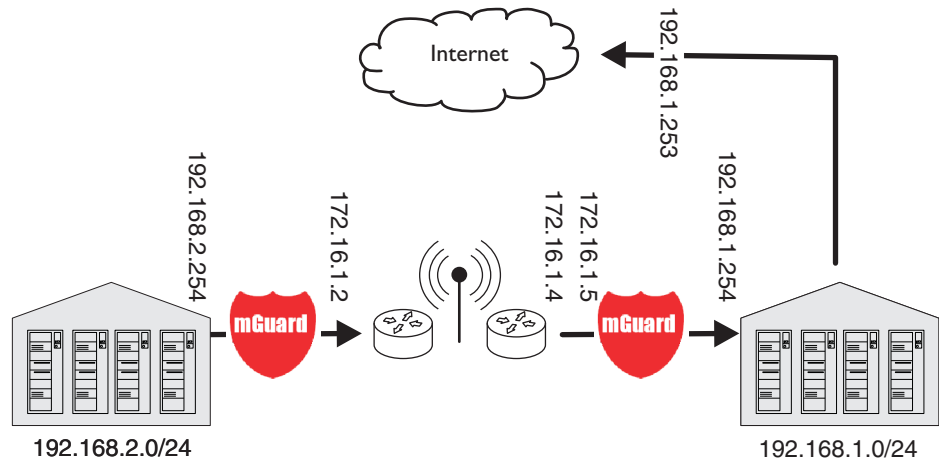
Bild 1-5 WLAN über VPN
