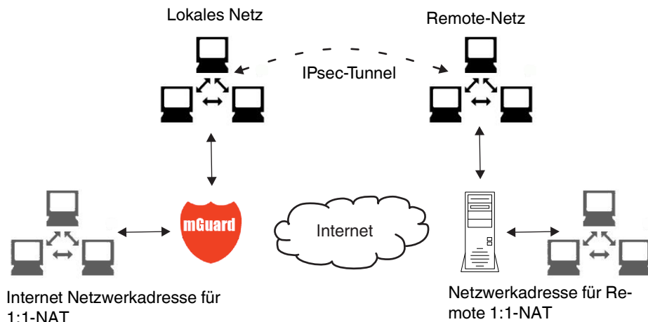
Bild 10-3 1:1-NAT
