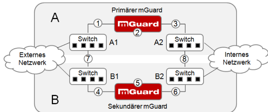
Bild 17-2 Mögliche Fehlerorte (1 ... 8)
